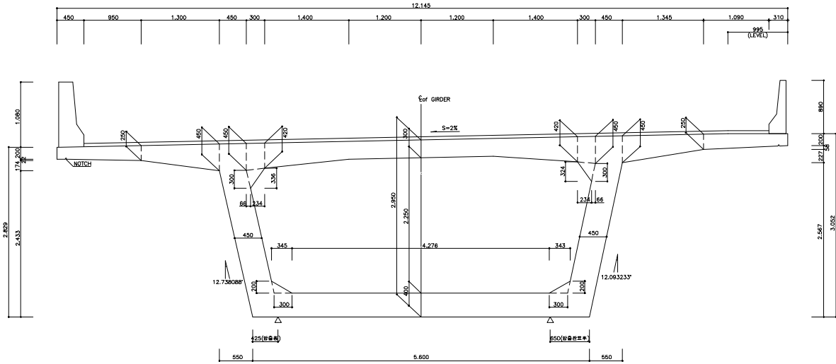
〈표준단면도 - 지점부〉
