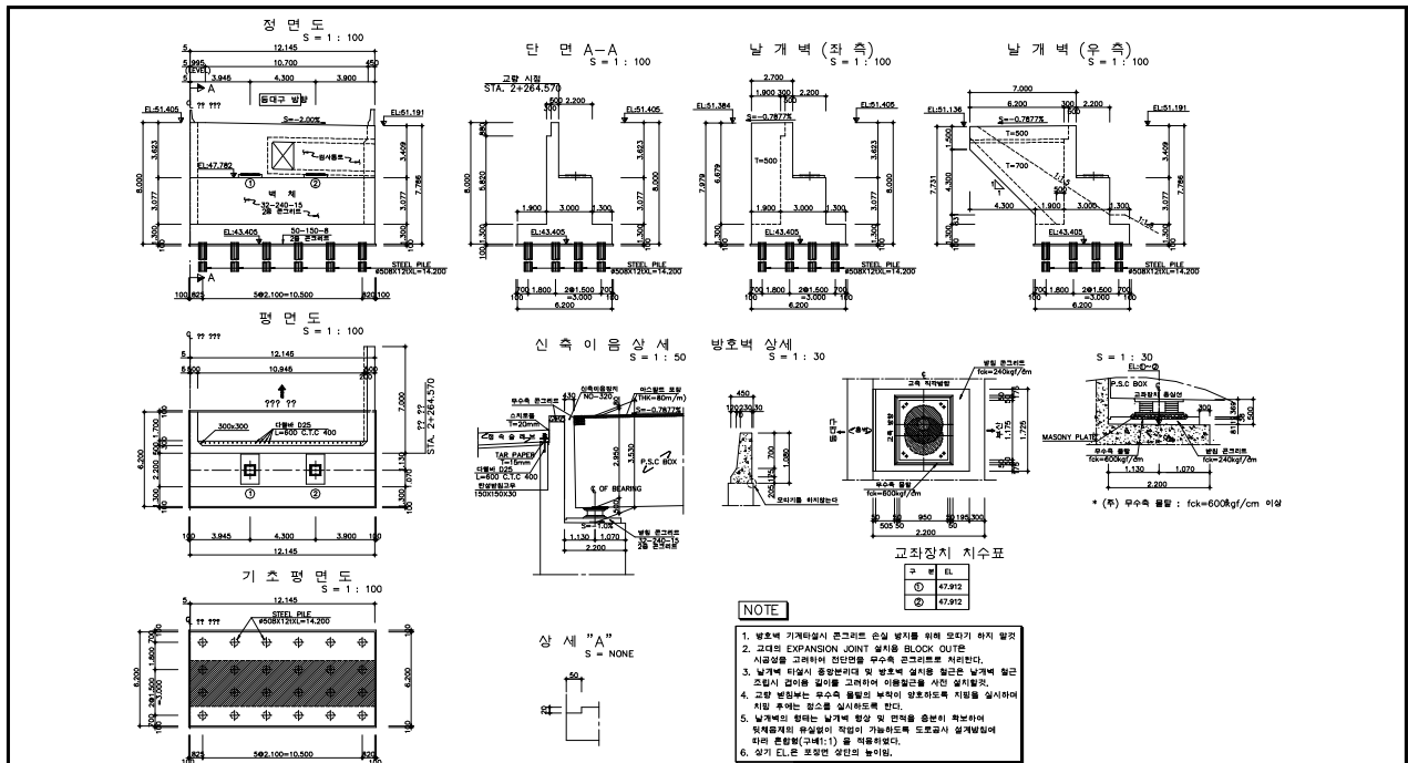
<교대 일반도 - 1>
