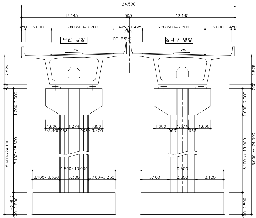
〈횡단면도〉
