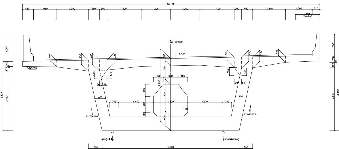
〈표준단면도 - 지점부(교각중심)〉
