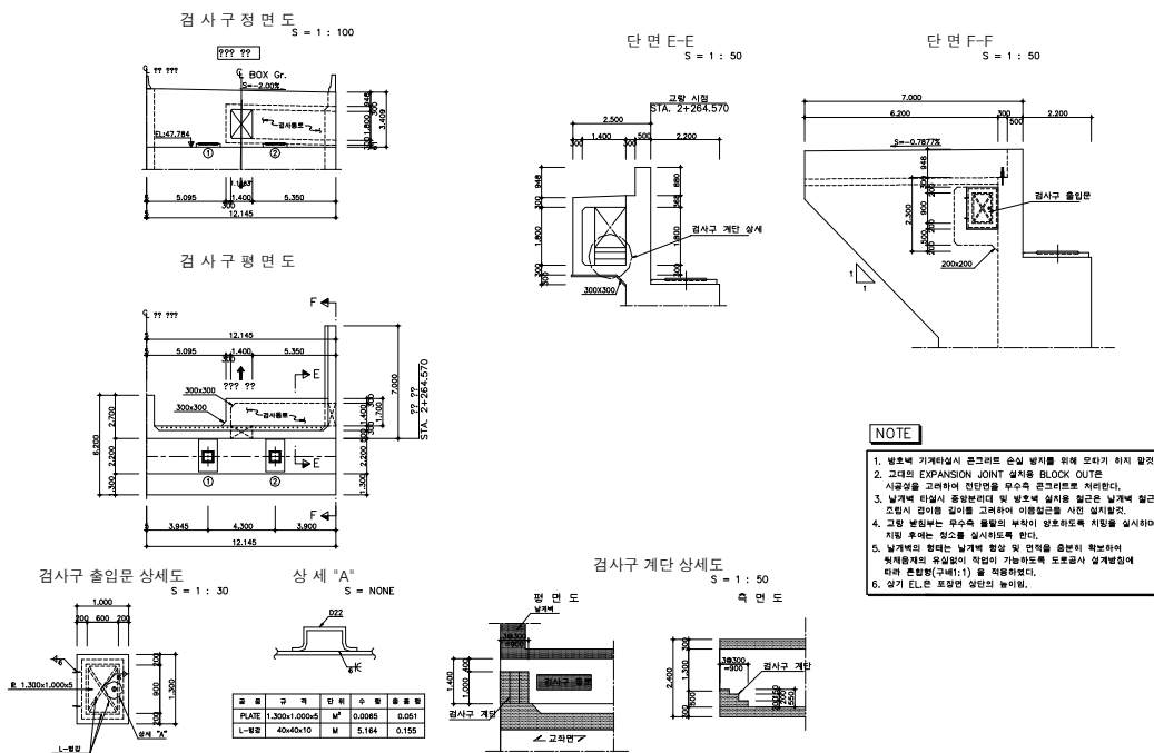
<교대 일반도 - 2>
