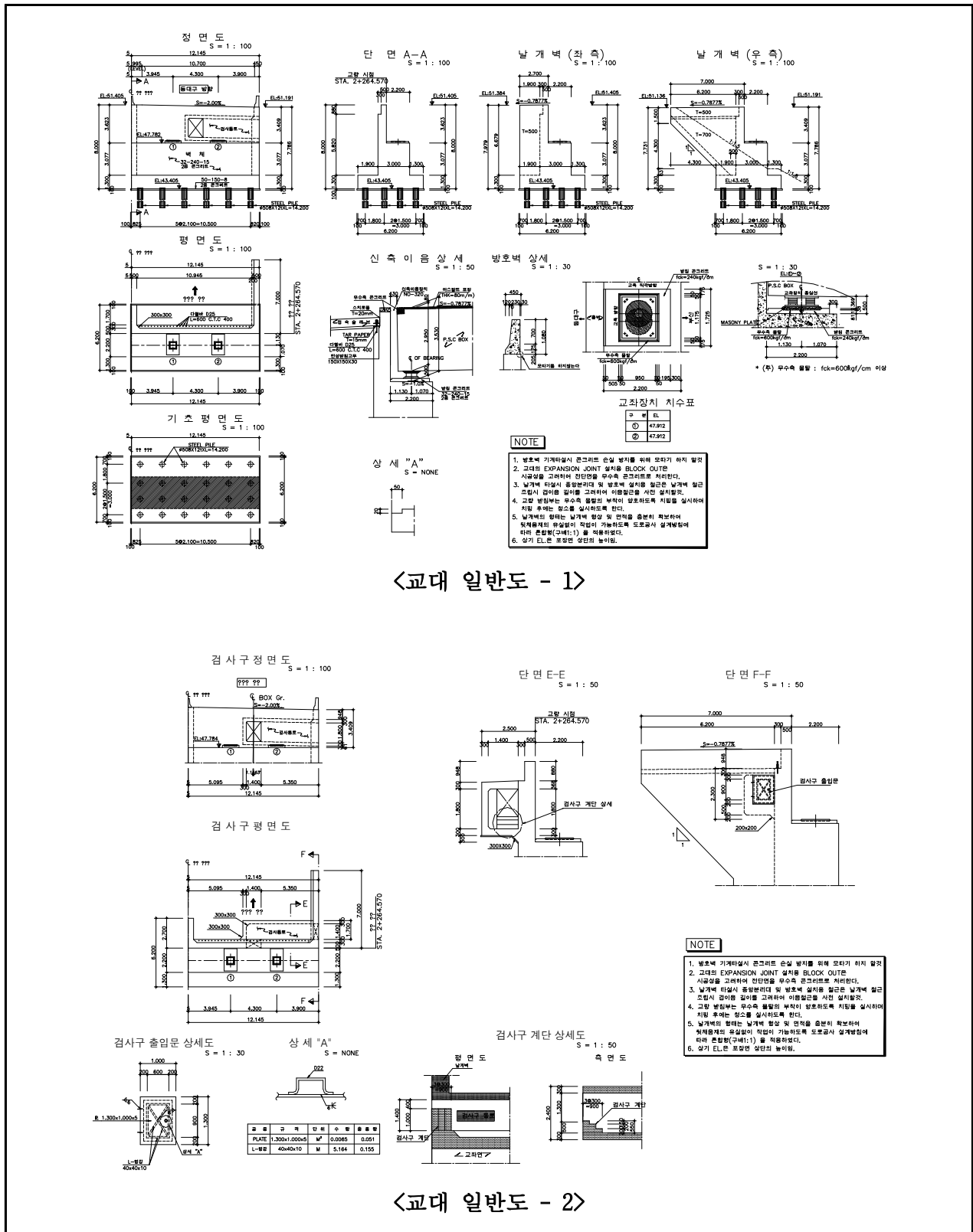
【그림 1.4.9】 금호강교(부산) 교대일반도
