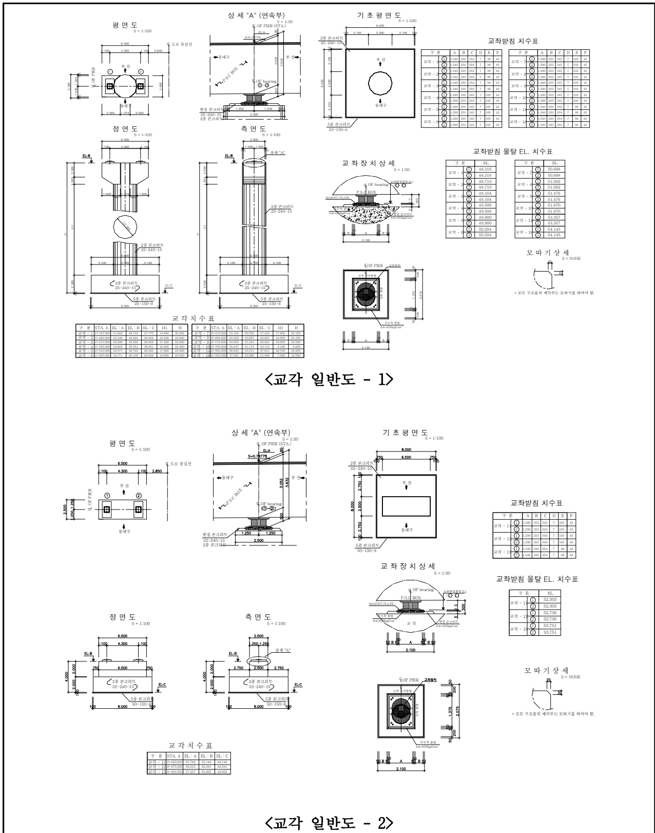
【그림 1.4.5】 금호강교(대구) 교각일반도
