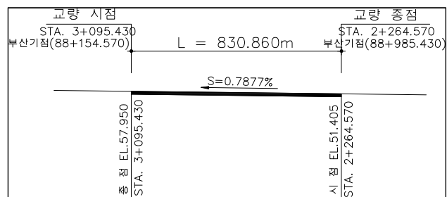
〈종단구배〉
